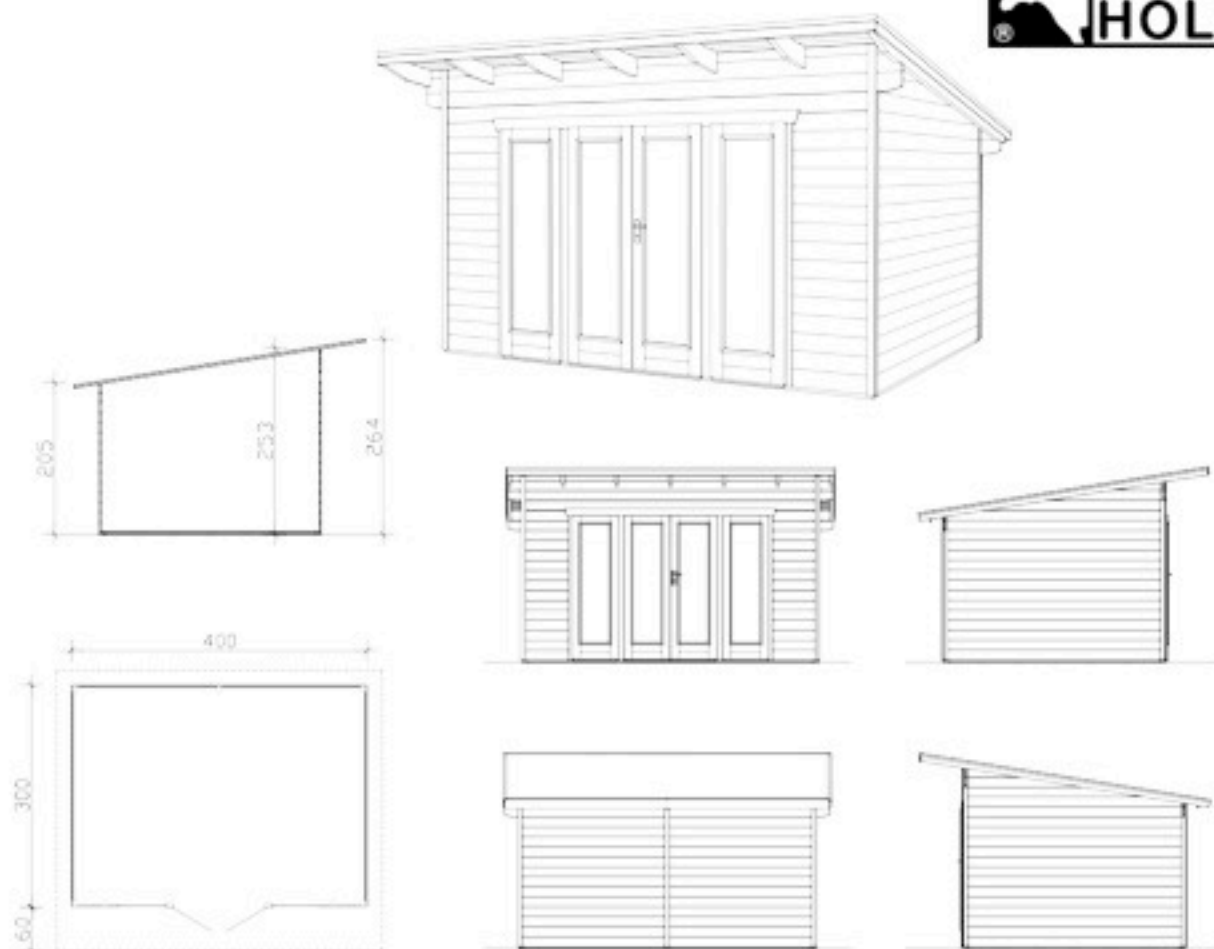
Grundriss, Schnitt und Ansichten M 1:100
